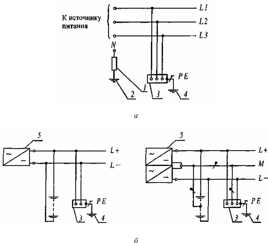
Рис. 1.7.4. Система IT переменного ( a ) и постоянного ( b ) тока. Открытые проводящие части электроустановки заземлены. Нейтраль источника питания изолирована от земли или заземлена через большое сопротивление:
